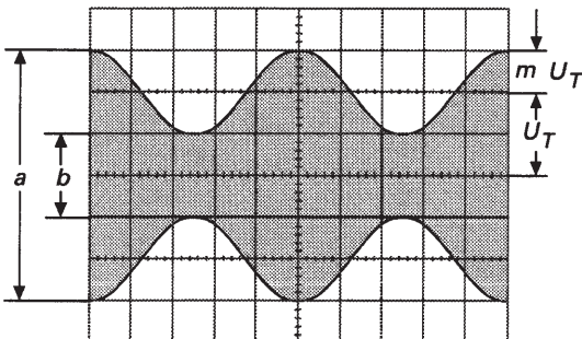
Figur 2: Amplitudenmodulierte Schwingung:
